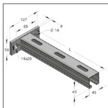
Konsola gotowa 45/45/2,0 poprzeczna
